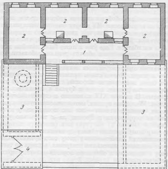
Рис. 42. Тип современного полутораэтажного дома (сел. Башлыкент Каякентского района):
