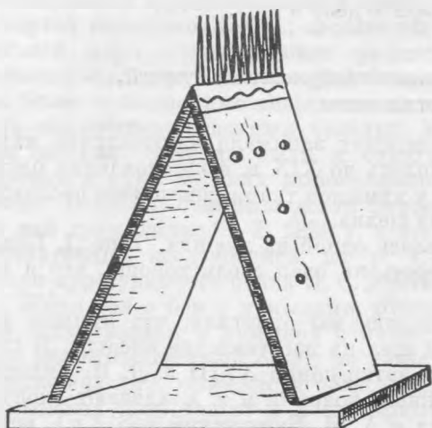
Рис. 11. Гребень для расчесывания шерсти
