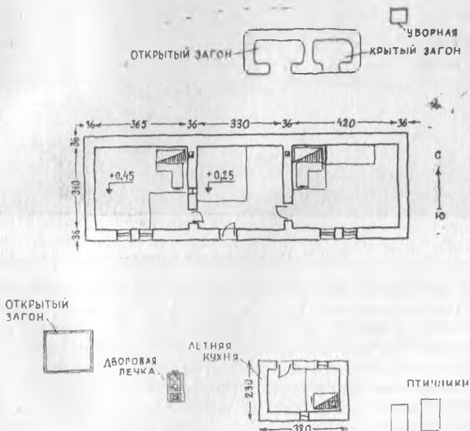
Рис. 6. Старое ногайское жилище; дом Алыпкашева в с. Нариман-аул; общий вид усадьбы и план усадьбы с планом дома.
