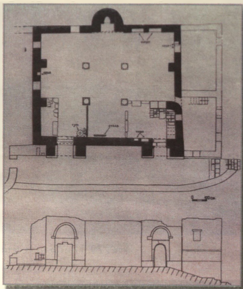
Рис. 27. Джума-мечеть. План и фасад. (сост. М.С. Гаджиев).
