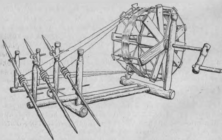
Прялка с колесом
