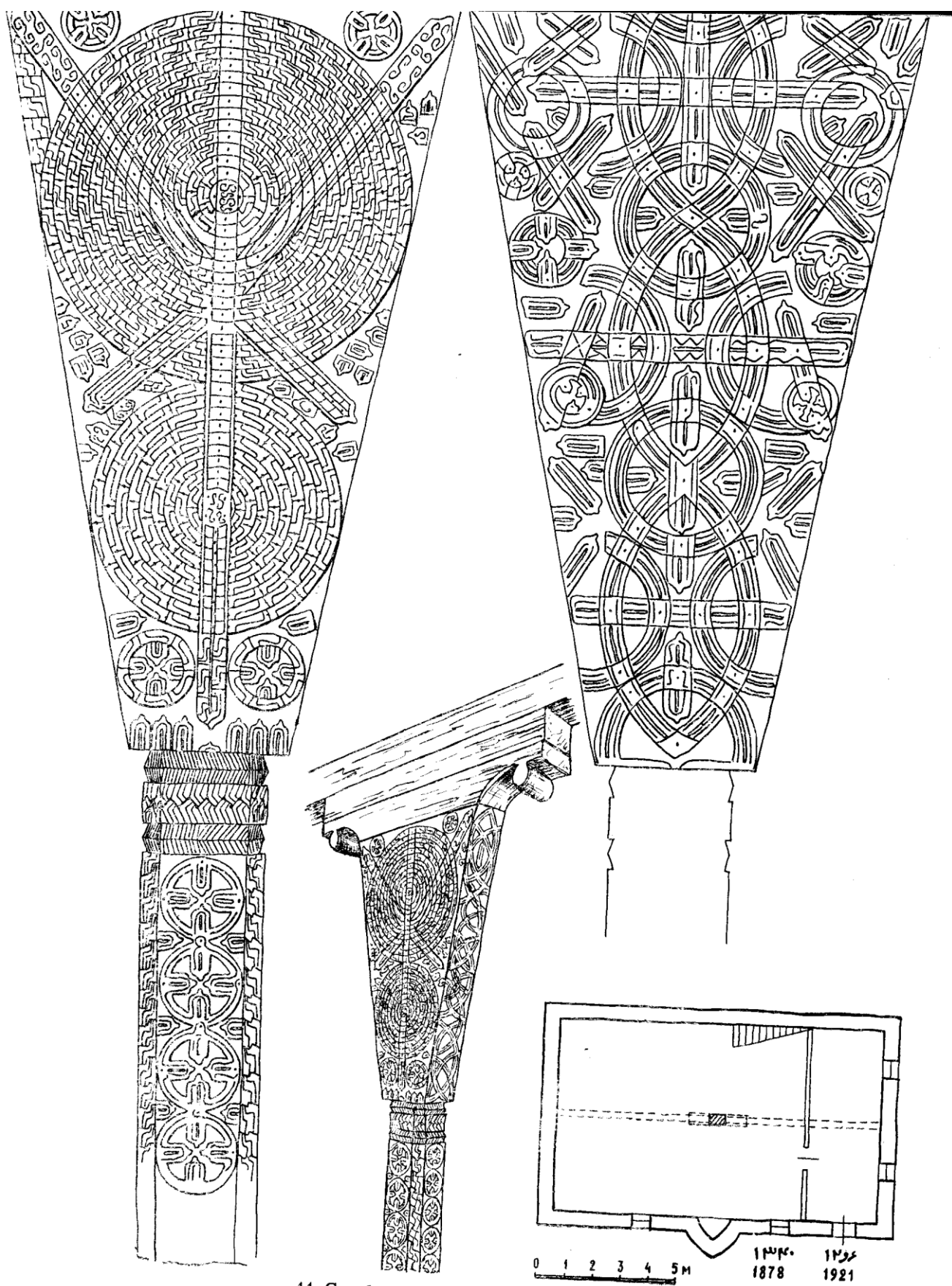
11. Столб мечети в сел. Турага Кайт. р-на.
