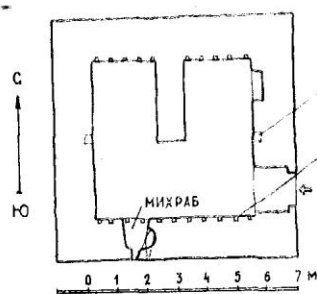
5. Развалины башни близ сел. Зубанчи Дах. р-на. а) Общий вид; б) план; в) бытовая ниша; г) михраб; д) проем входа.
