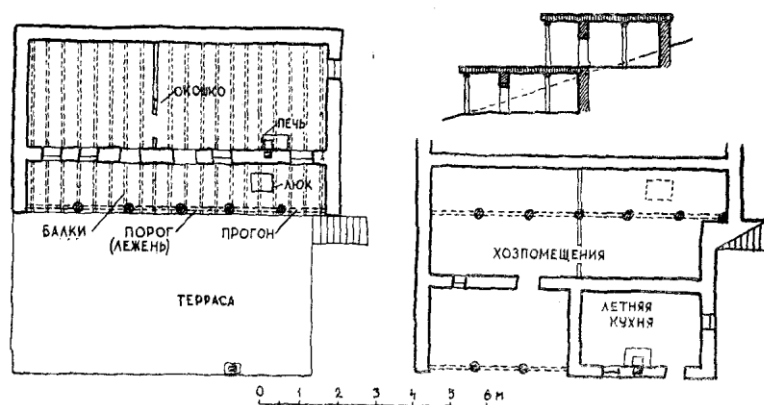
1. Дом Магомедова в сел. Ниж. Ишкарты Буйн. р-на.
