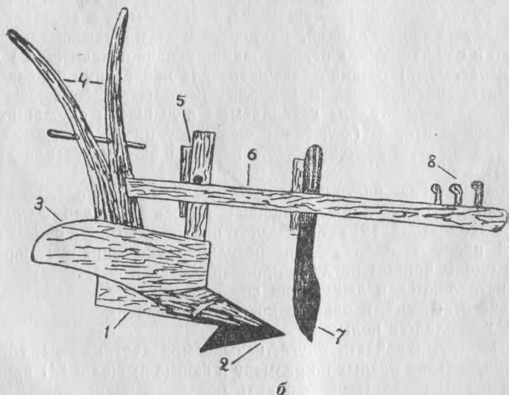
Рис. 1. Кумыкский плуг-сабан для двух пар волов: а—общий вид; б—рабочая часть.
