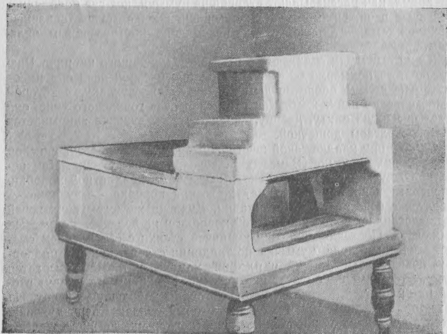
Рис. 19. Современная комнатная печь северных кумыков
