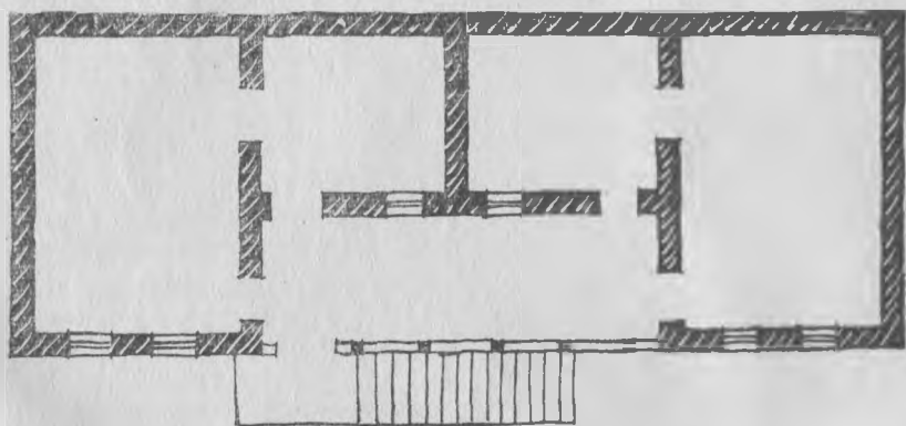
Рис. 13. План двухэтажного „п“-образного дома: а—план нижнего этажа; б—план верхнего этажа.
