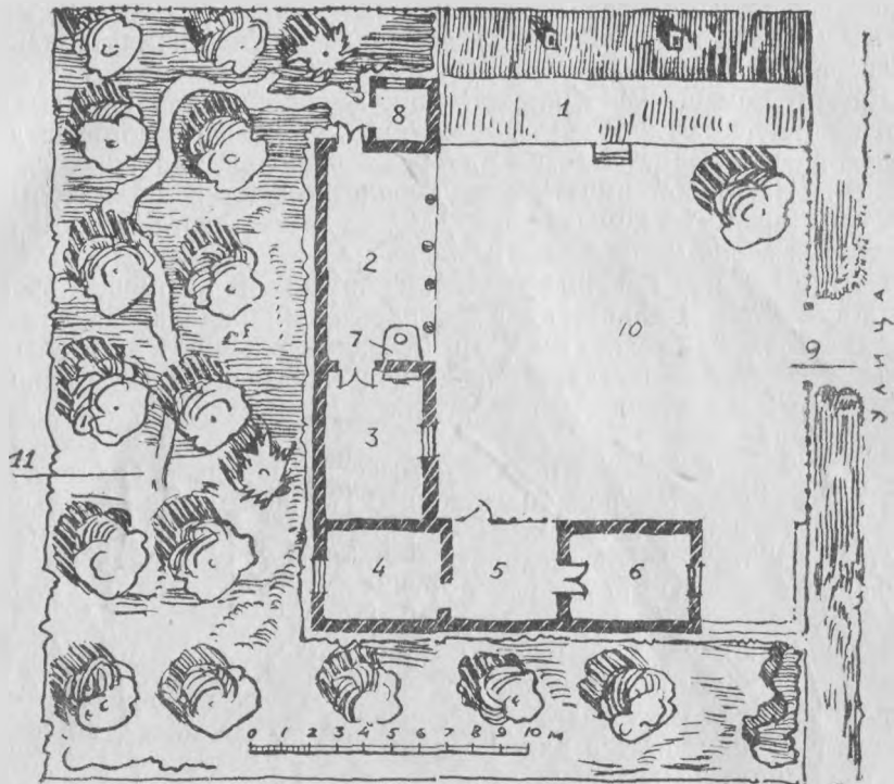
Рис. 16. План новой усадьбы: 1—жилой дом; 2—летний хозяйственный навес; 3—летняя кухня; 4—помещение для скота; 5—навес для скота; 6—помещение для скота; 7—печь 8—курятник; 9—ворота; 10—двор; 11—сад.
