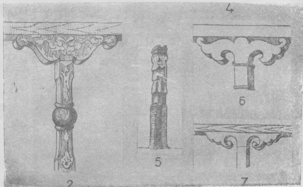
Рис. XIX. Центральные столбы в горах, в сс. Кала-Корейш и Кубачи.
